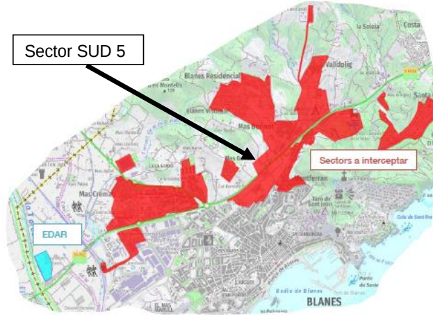
Figura 3. Sectors a interceptar i ubicació EDAR.
